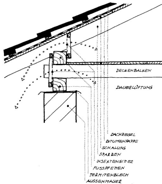
DACHDETAIL DOPPEL FUSSPFETTE MIT DAUERLÜFTUNG MASSSTAB 1:10
