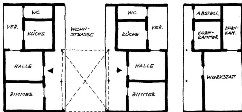
GRUNDRISS II
